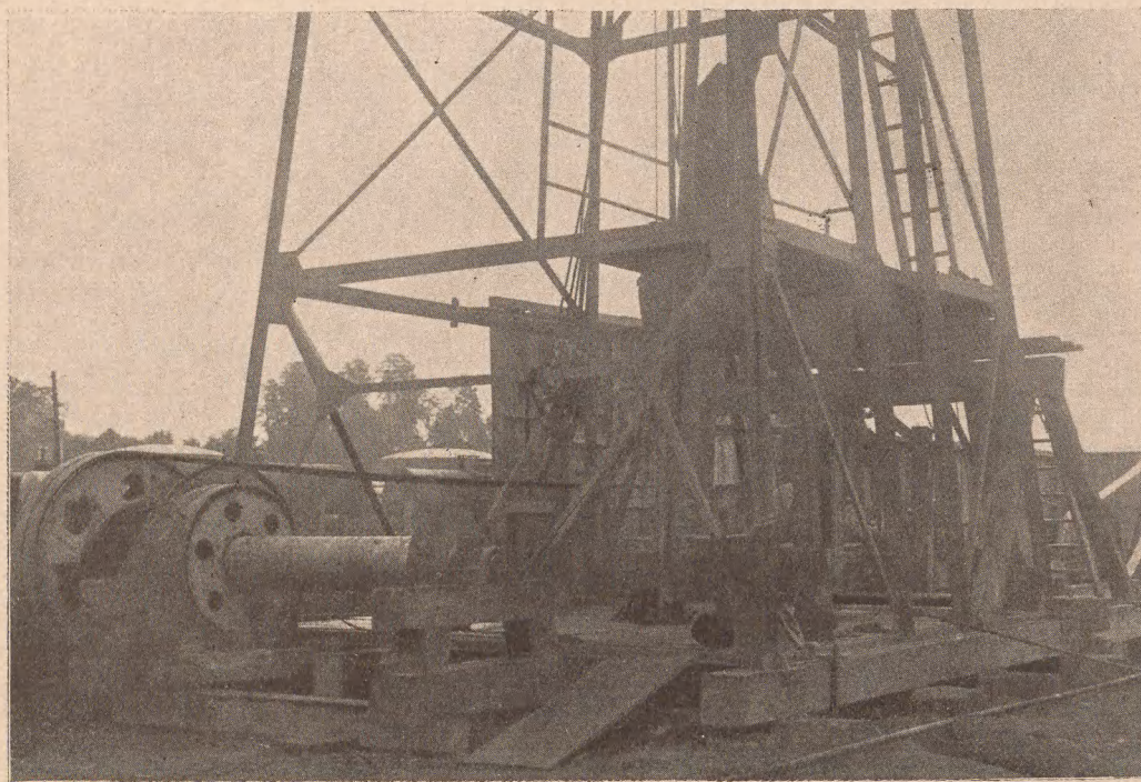
Widok na bę- ben świdrowy i dolną część wieży.
