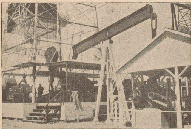
Żuraw pompowy „Emsco“, w głębi żuraw rotacyjny „Emsco“.
